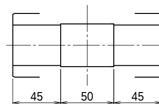
出力軸内部詳細 (尺度 1/2.5)
