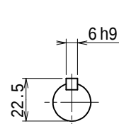
入力軸
