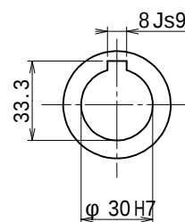
出力軸
