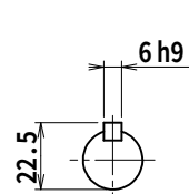
入力軸
