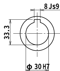
出力軸
