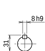
入力軸
