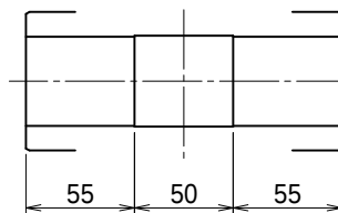
出力軸内部詳細
