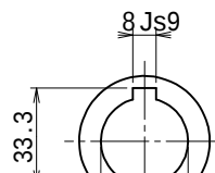
出力軸
