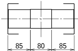
出力軸内部詳細 (尺度 1/6)
