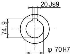
出力軸 (尺度 1/6)
