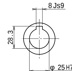
出力軸 (尺度 1/2)
