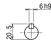
入力軸 (尺度 1/2)
