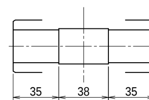
出力軸内部詳細 (尺度 1/2)
