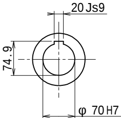
出力軸 (尺度 1/6)
