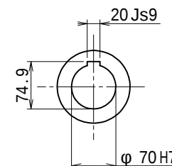
出力軸 (尺度 1/6)
