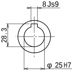
出力軸 (尺度 1/2)
