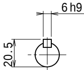
入力軸 (尺度 1/2)
