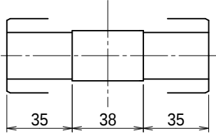
出力軸内部詳細 (尺度 1/2)
