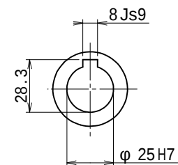
出力軸 (尺度 1/2)
