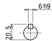
入力軸 (尺度 1/2)
