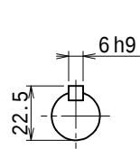
入力軸 (尺度 1/2)
