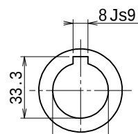
出力軸 (尺度 1/2)
