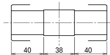
出力軸内部詳細 (尺度 1/2)
