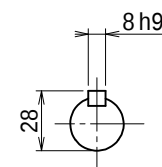
入力軸 (尺度 1/2.5)
