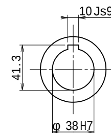
出力軸 (尺度 1/2.5)
