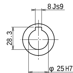
出力軸 (尺度 1/2)
