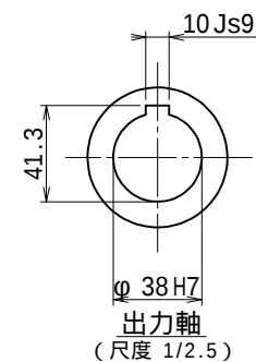
出力軸内部詳細 (尺度 1/2.5)
