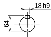
出力軸
