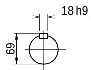
出力軸
