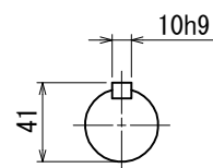
出力軸 (尺度 1/3)
