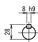
入力軸
