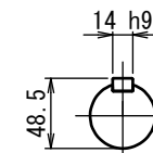
出力軸
