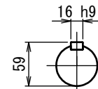
出力軸
