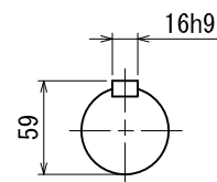
出力軸 (尺度1/3)
