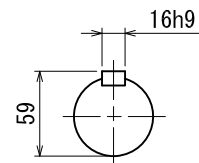
出力軸 (尺度1/3)
