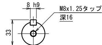
出力軸
